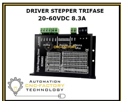
DRIVER MOTORE STEPPER TRIPOLARE 8A 20-60V DC INPUT
